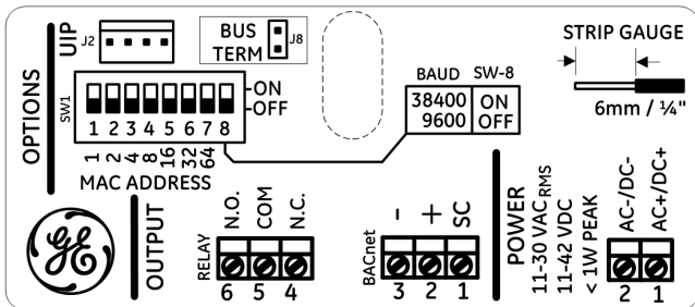
BACnet Wiring
