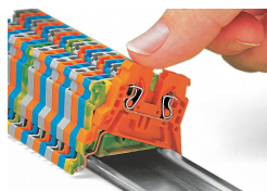
Montaż złączki listwowej na szynie DIN 35
