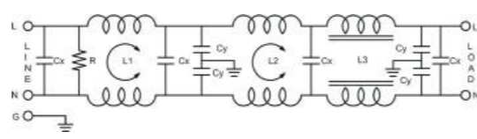
电气原理图(Electrical Schematic) : 42
