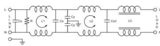
电气原理图(Electrical Schematic) : 43
