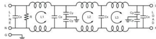
电气原理图(Electrical Schematic) : 42
