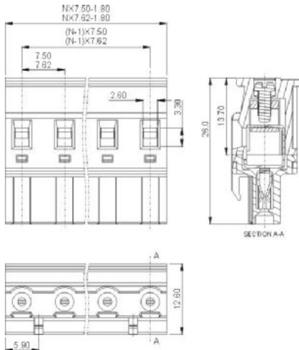
2EDGKA-7.5 2EDGKA-7.62
