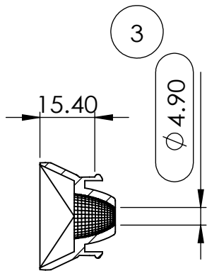
剖面图 A-A
