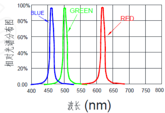
波长特性
